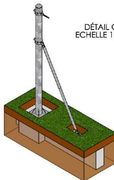
Poteau 220x11cm sur platine et jambe de force acier galvanisé à chaud (différentes finitions possibles)
